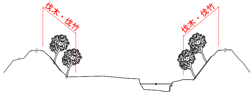
標準断面図 (宮川内谷川)
